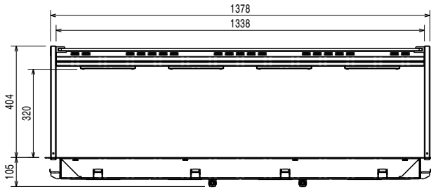
Zij aanzicht
